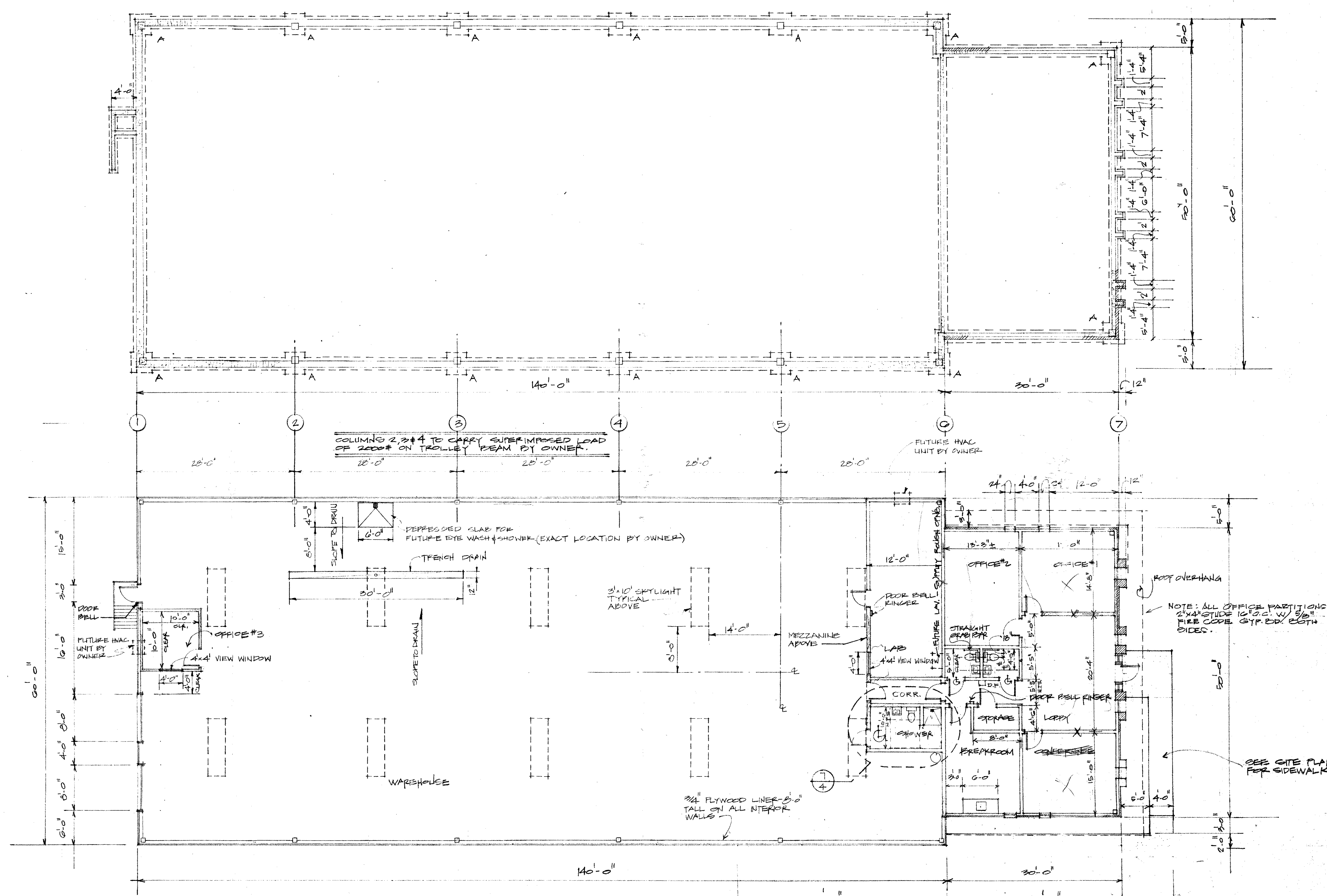
1 PLAN 2 SCALE: 1/8" = 1'-0"
